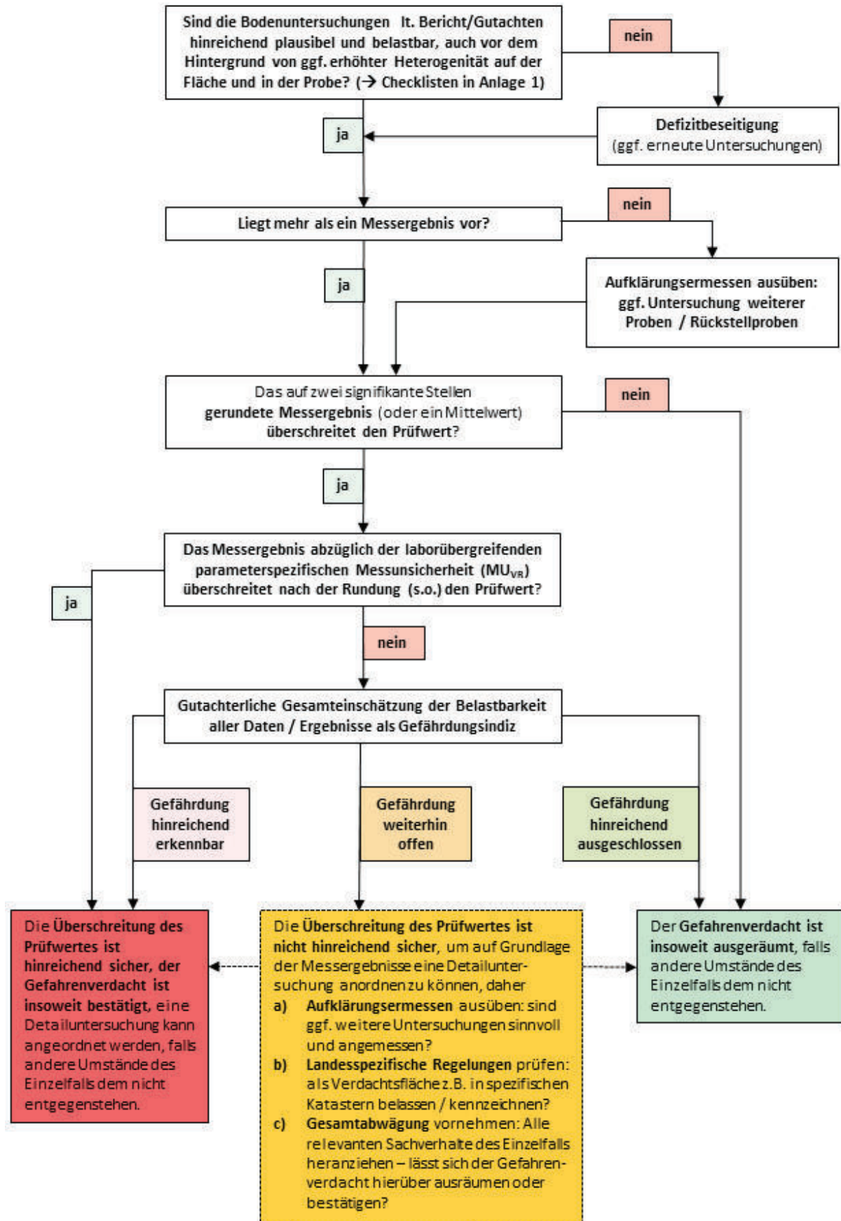
Abbildung 1: Empfehlungen zum Einbezug der Mess- und Ergebnisunsicherheit bei der Beurteilung von Messergebnissen im Nahbereich von Prüfwerten im Rahmen der Orientierenden Untersuchung.
