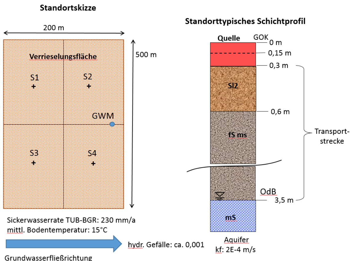
Abb. 58: Standortskizze und standorttypisches Schichtprofil für das Fallbeispiel 2
