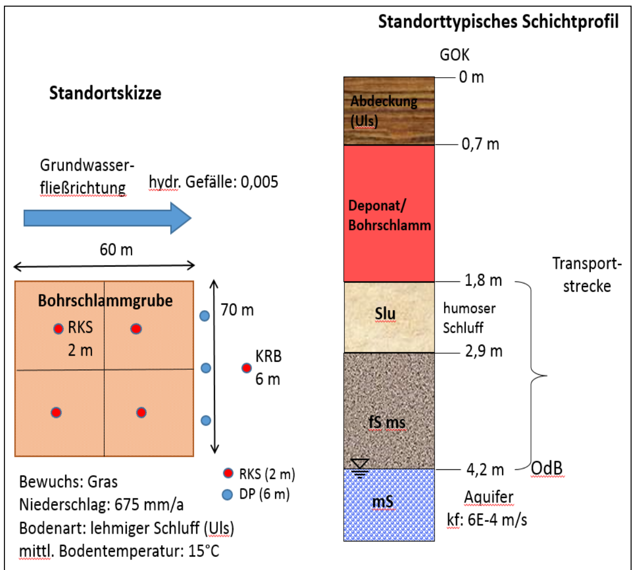
Abb. 64: Standortsskizze und standorttypisches Schichtprofil für Fallbeispiel 3 (Bohrschlammgrube)
