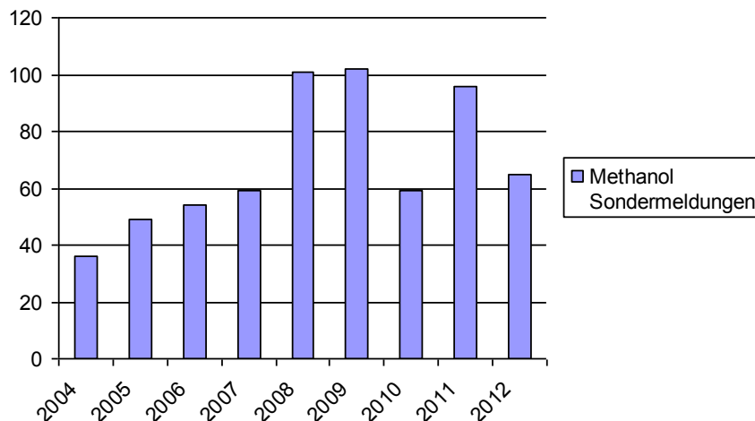
Abb. 7: Gefundene Methanolangebote 2004-2012
