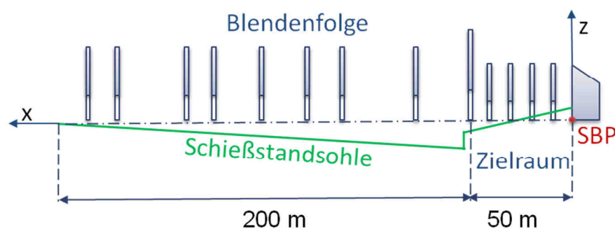
Abbildung 5 Skizze zum Bezugssystem im Schießstandtyp A, Darstellung in der Schießstandmittelebene Schießrichtung von links nach rechts Absicherungsgrad III
