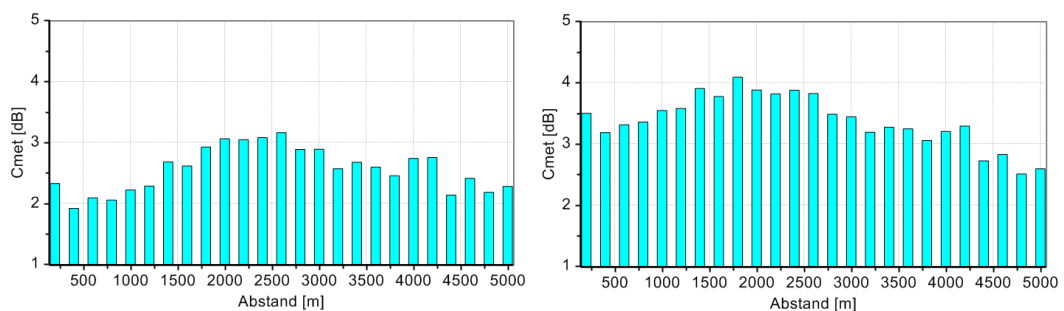
Abbildung 19 Abstandsabhängigkeit der meteorologischen Korrektur nach Fehler! Verweisquelle konnte nicht gefunden werden. für die Richtungen Norden (links) und Süden (rechts)
