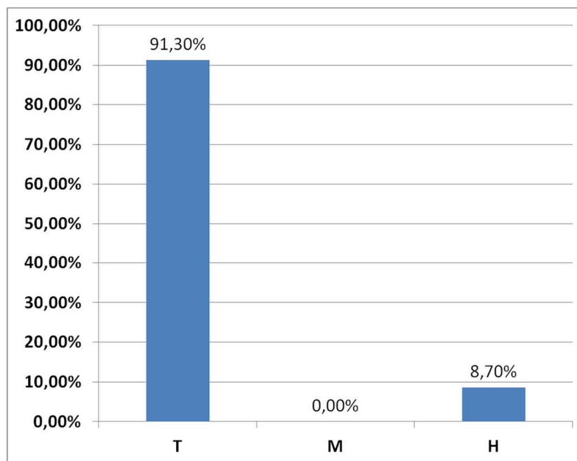
Abbildung 10 Relative Verteilung der Anschlagklassen bei der Annahme einer gleich häufigen Nutzung der Betriebssituationen auf einem D-Stand, Dunkelheitsschießen
