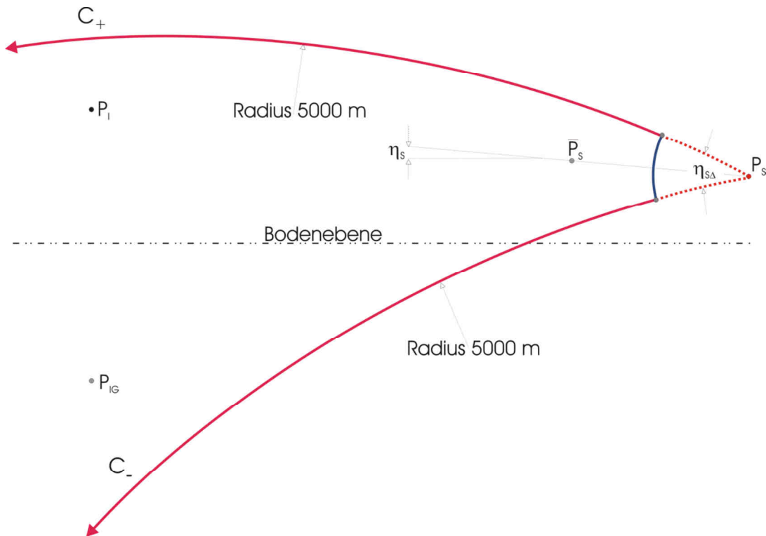
Abbildung 18 Vertikaler Schnitt der Ausbreitungssituation
