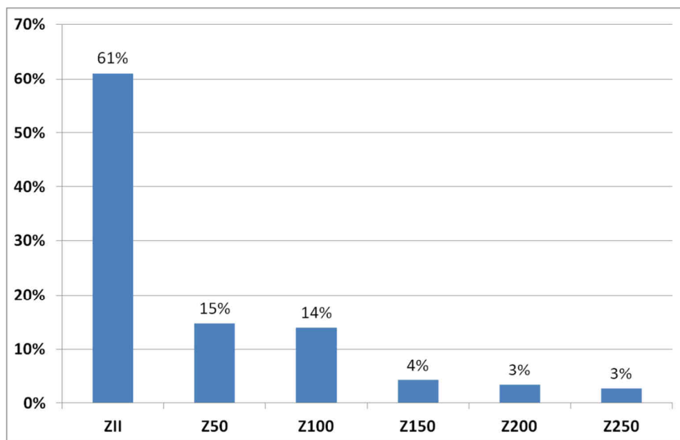
Abbildung 7 Relative Verteilung der Schusszahlen auf die Abstandszonen bei der Annahme einer gleich häufigen Nutzung der Betriebssituationen auf einem A-Stand, Helligkeitsschießen
