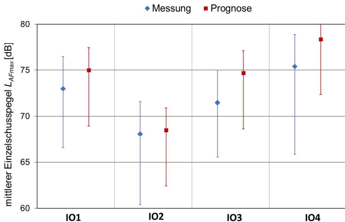
8 Abbildung 28 Vergleich von Messung und Prognose unter Berücksichtigung der Vertrauensbereiche 9 Grundlage der Prognose sind die Werte nach Tabelle 15 (Gelände) 10
