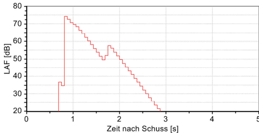
Abbildung 26 L_{AF} am Immissionsort IO1
