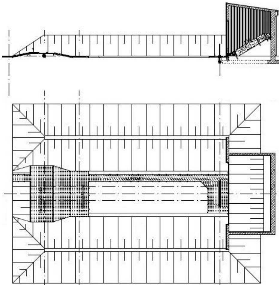
Abbildung 4 Schießstand Typ D 25 m mit Absicherungsgrad I
