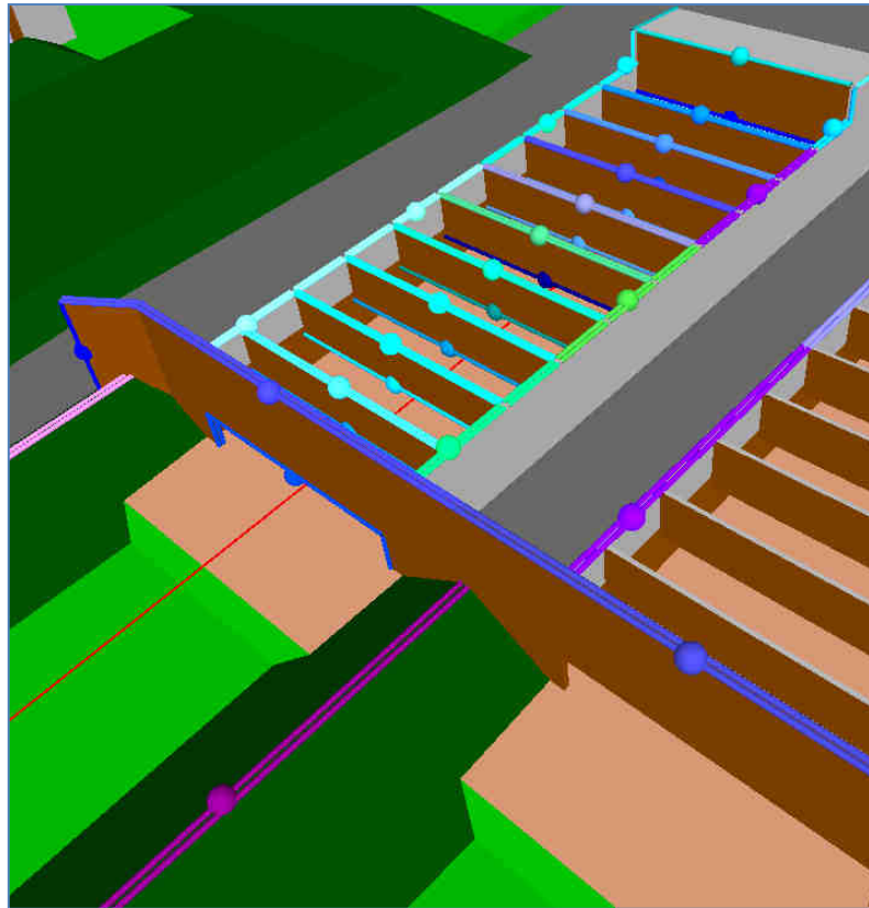
Abbildung 23 Zuordnung einzelner Kantensegmente zu Beugungsersatzquellen
