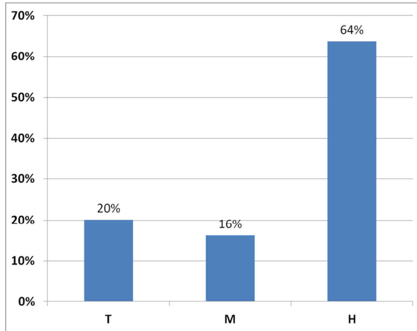
Abbildung 8 Relative Verteilung der Anschlagklassen bei der Annahme einer gleich häufigen Nutzung der Betriebssituationen auf einem A-Stand, Helligkeitsschießen
