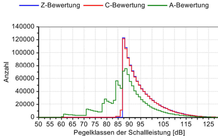
Abbildung 25 Anzahl der Teilersatzquellen in 1-dB-Klassen des immissionswirksamen Schallleistungspegels für die Ersatzquelle
