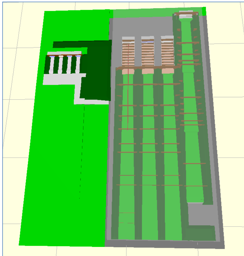
Abbildung 20 Gesamtanlage mit Schießstandkörper (grau) und Schusslinie (rot)
