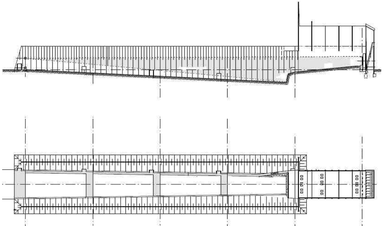
Abbildung 2 Schießstand Typ A 250m mit Absicherungsgrad I
