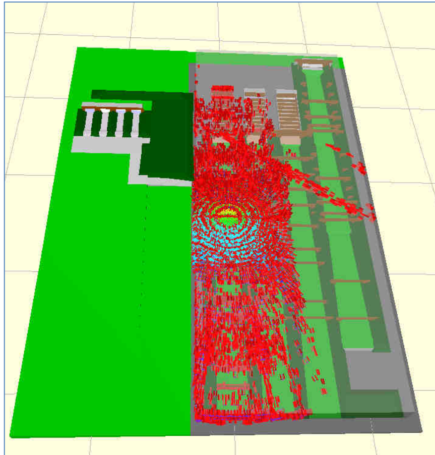
Abbildung 24 Darstellung der Zelte, die nach Anwendung des Schießstandquellmodells bei diesem Beispiel auf dem Schießstandkörper als Grundlage für die Bildung der Teilersatzquellen dienen
