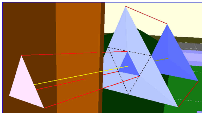
Abbildung 22 Dynamische Strahlaufteilung an einer Kante
