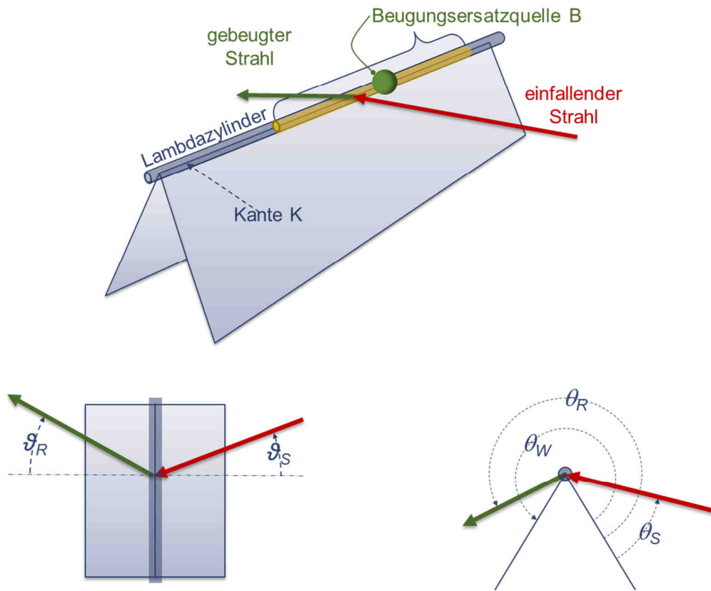
Abbildung 16 Zur Definition der Winkel bei der Beugung oben: Kante K mit den sie bildenden Flächen des Grundkörpers, Beugungsersatzquelle B mit dem ihr zugeordneten Bereich der Kante, dem einfallenden Strahl und einem ausfallenden Strahl unten links: Aufsicht unten rechts: Schnitt quer zur Kante
