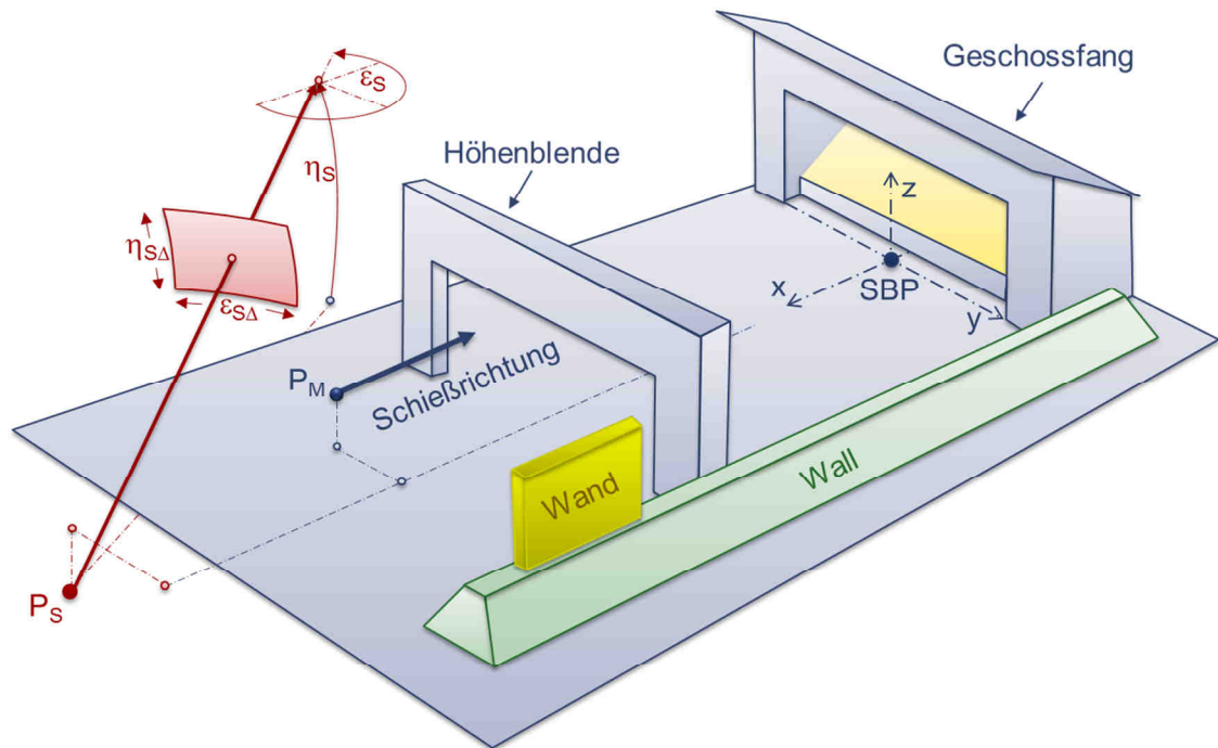
Abbildung 15 Skizze eines Schießstandes mit grundlegenden Elementen und Kennzeichnung der geometrischen Eigenschaften einer Teilersatzquelle
