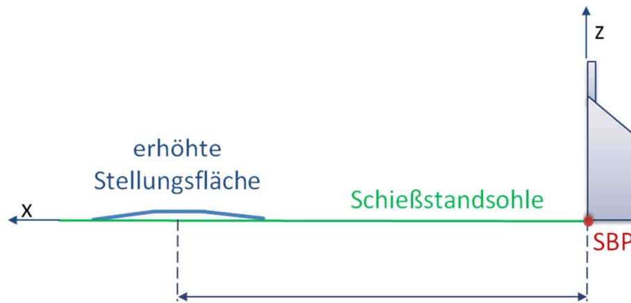
Abbildung 6 Skizze zum Bezugssystem im Schießstandtyp D Darstellung in der Schießstandmittelebene Schießrichtung von links nach rechts
